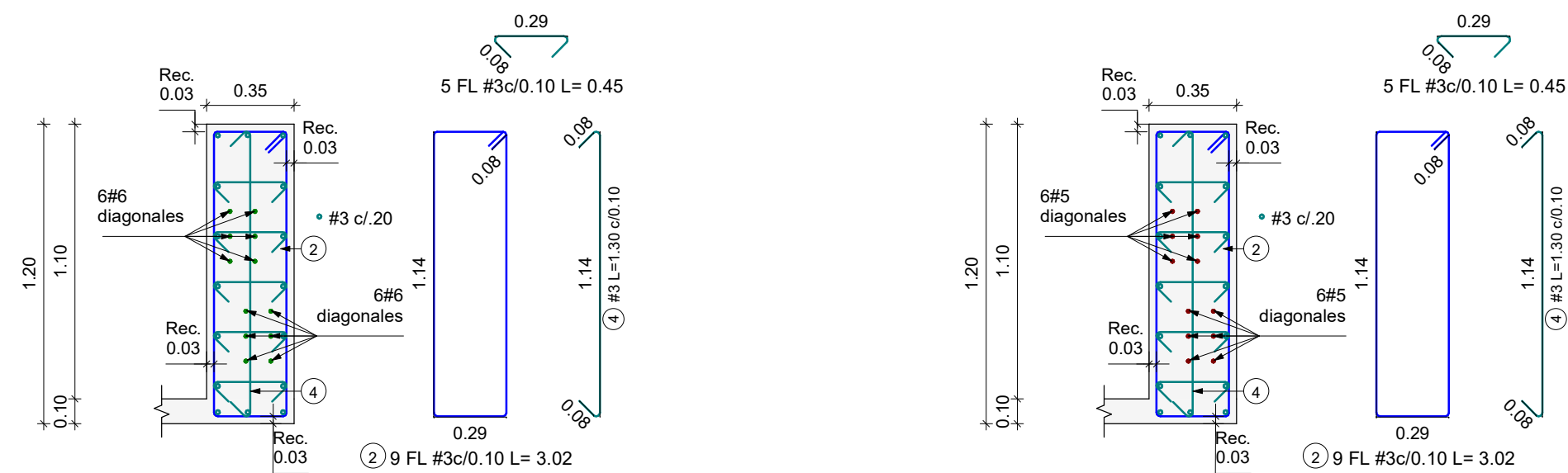
CORTE 1 - 1 VIGA DE ACOPLE TIPO 2 e=0.35 Escala 1 : 25
